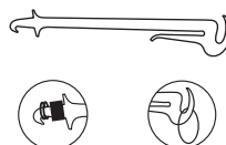
RP23489 Plumbers Hook - Seat, Spring & Spout O-Ring Removal Tool Gancho de Plomero-Asiento, Resorte y Herr. para Sacar Anillo "O" del Tubo de Salida
